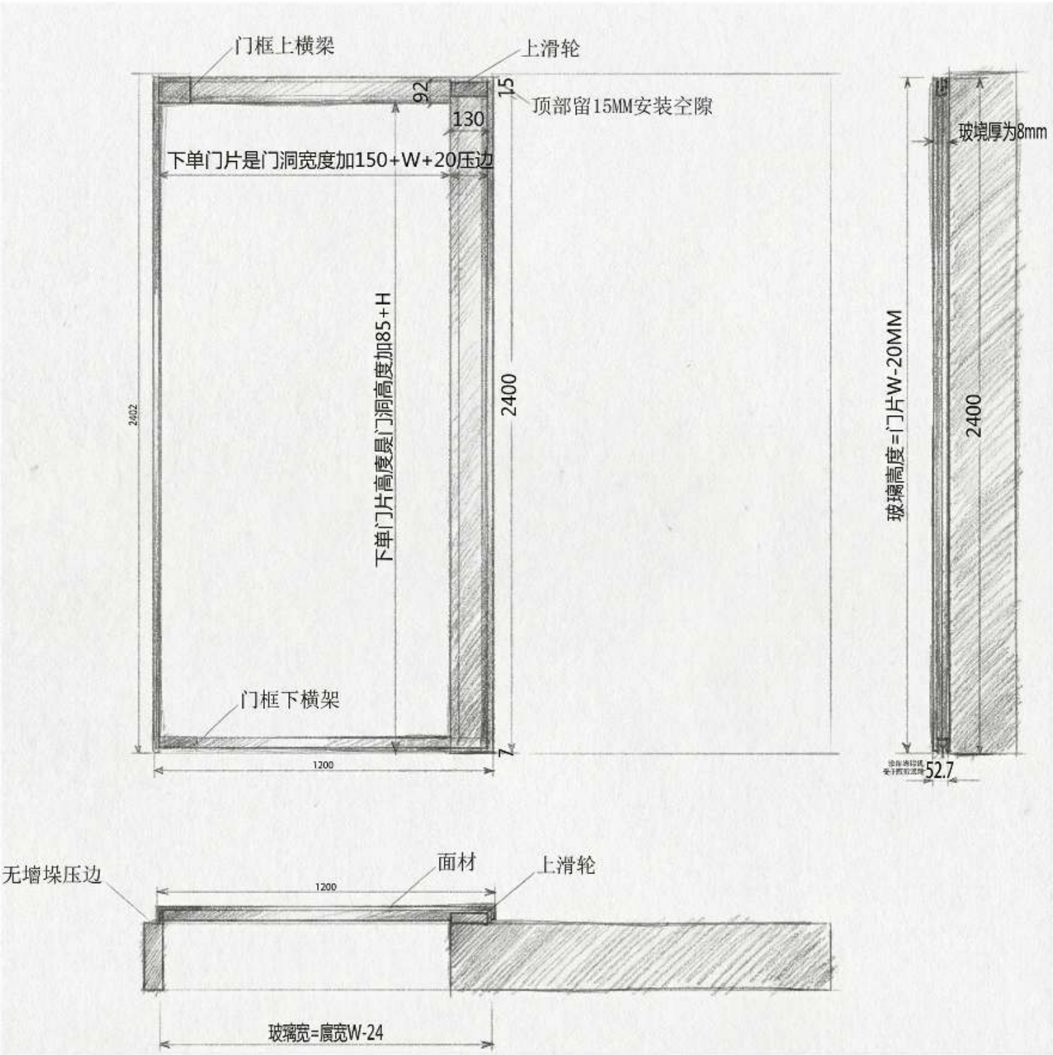
产品技术图
