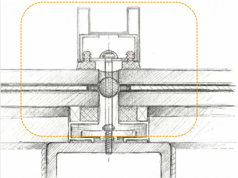
典型明框做法
