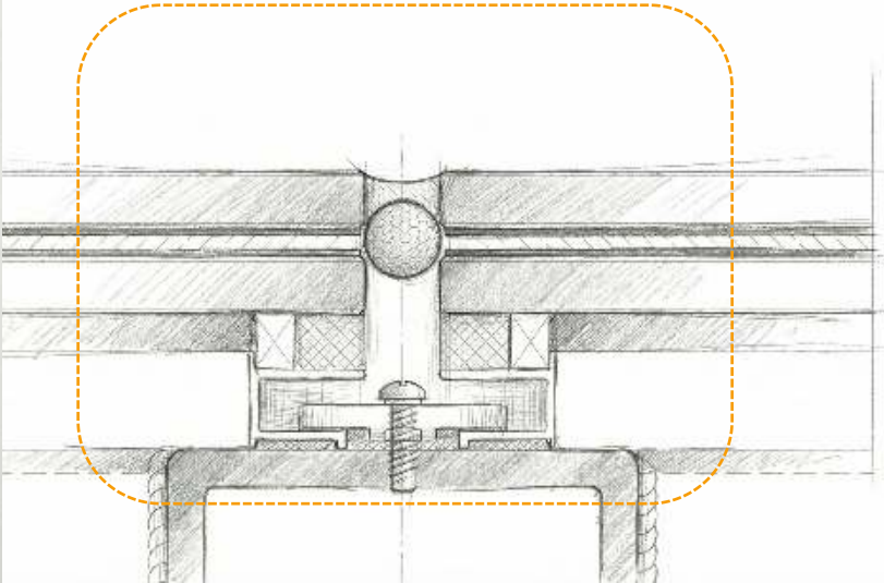
典型隐框做法
